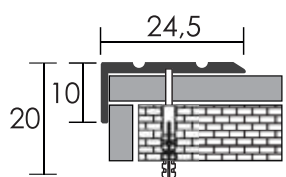
Pravouhý schodový profil - vrtaný, hliník
