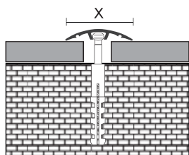
Přechodová lišta se skrytým kotvením, hliník
